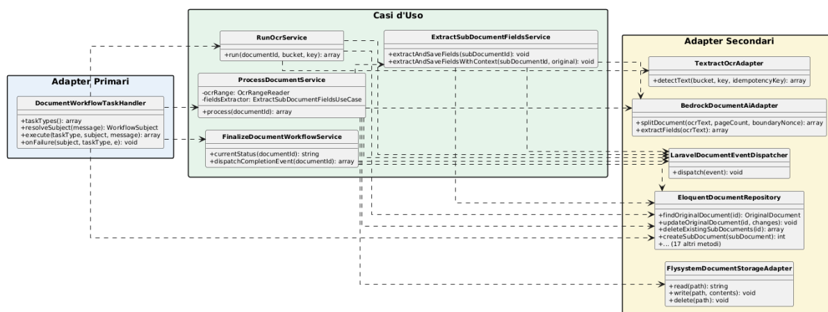
Figura 9: Diagramma classi parziale — Flusso di elaborazione OCR/AI
